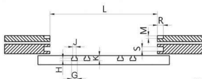
Ejector
