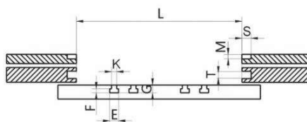
Ejector
