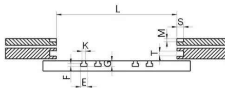
Ejector
